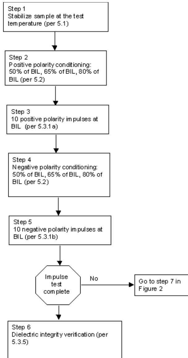
Figure 1—Impulse BIL test
